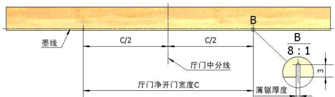
图 5-2 在井道底部做同样一副样板架，其上下样板架各部分垂直投影线应一致。
