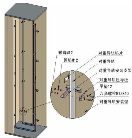
对重导轨与导轨支架安装
