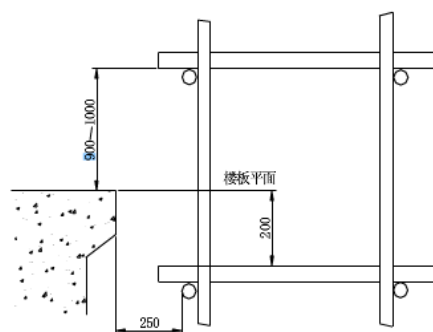
图 5-5 层门入口处样板
