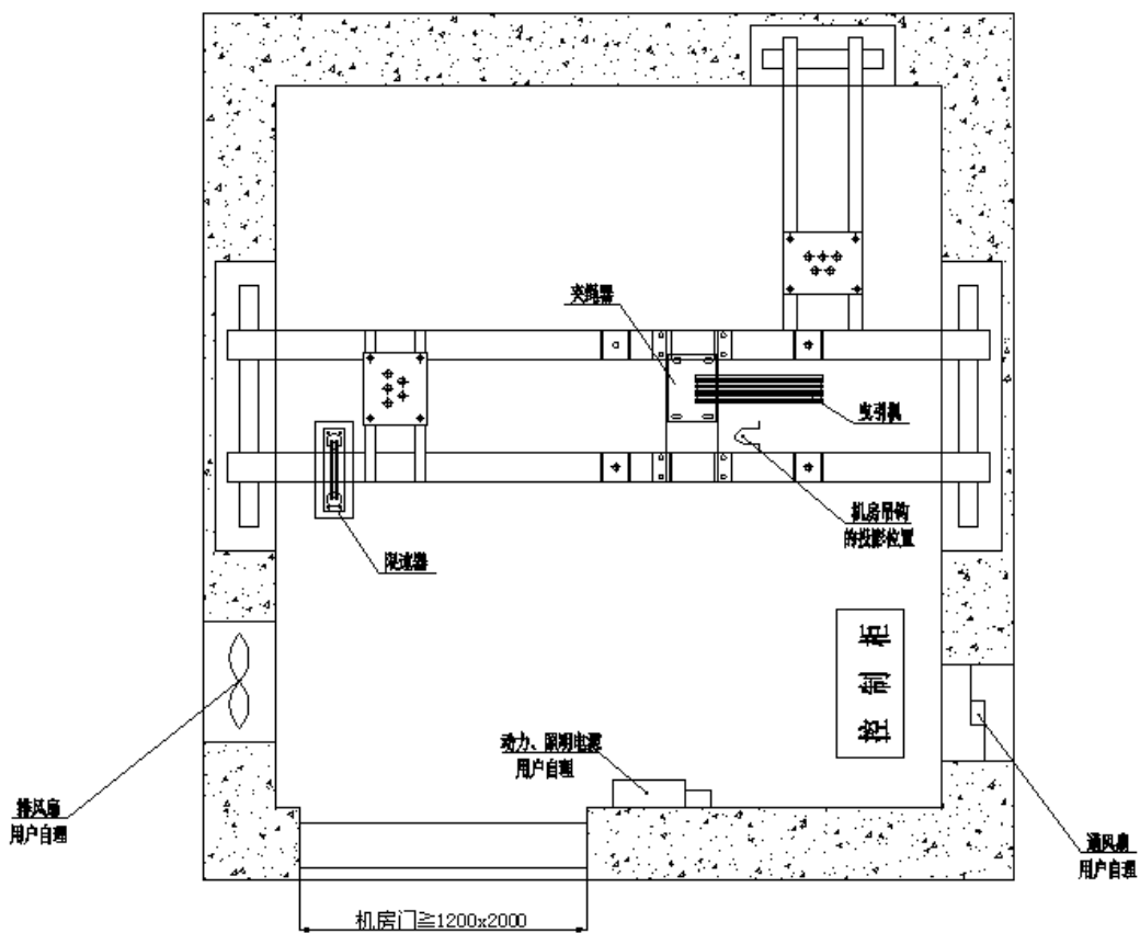
图 1-3 有机房曳引比 2:1
