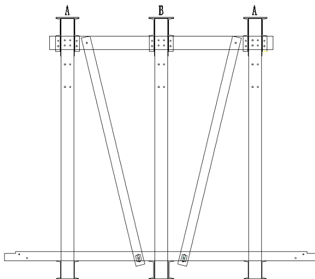
图 11-3 四导轨（AB）和六导轨（ABA）载货电梯（适用于中高吨位电梯）
