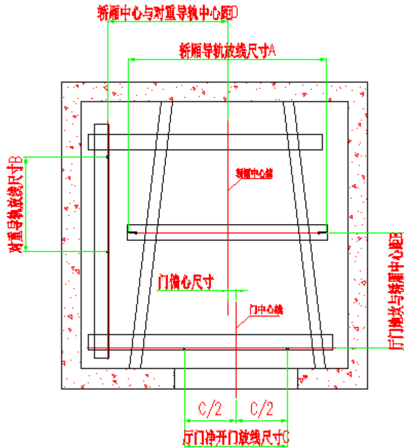
图 5-4 本图为对重侧置
