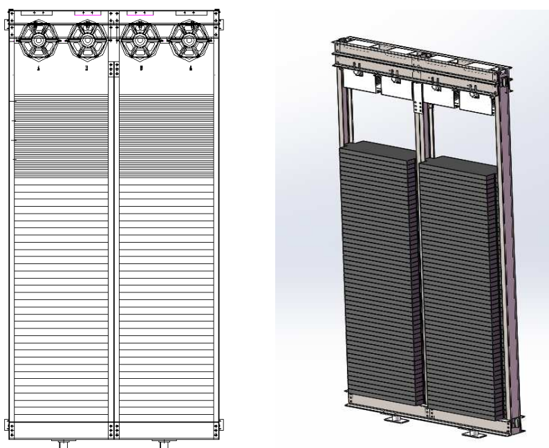
图 10-4 4:1 对重装置（AA 或 BB）与 8:1 对重装置（AABB）适用于中吨位和高吨位货梯
