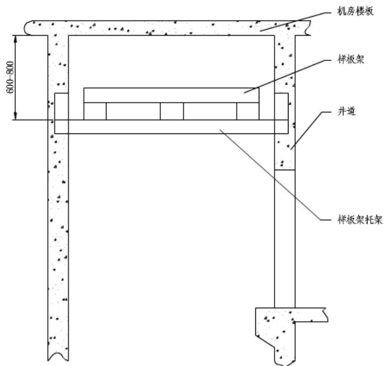
图 5-6 顶层楼板处样板
