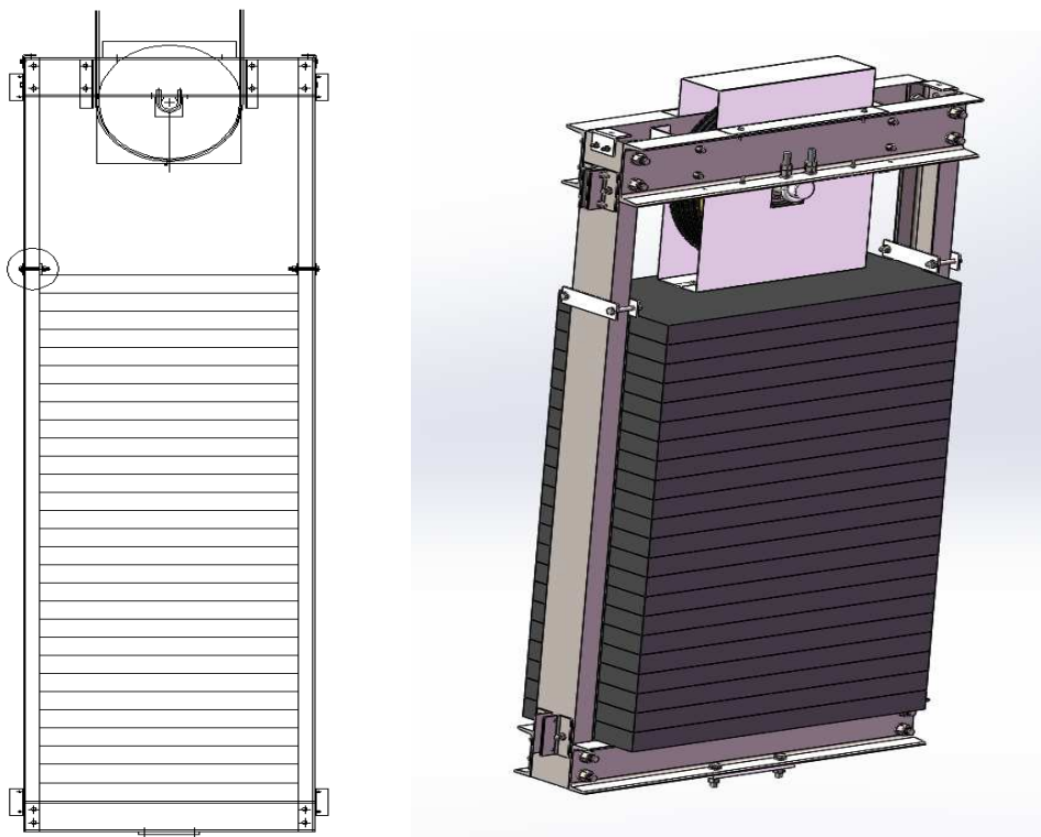
图 10-3 2:1 对重装置（适用低吨位货梯）
