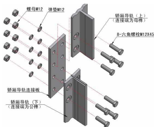
轿厢导轨对接示意图
