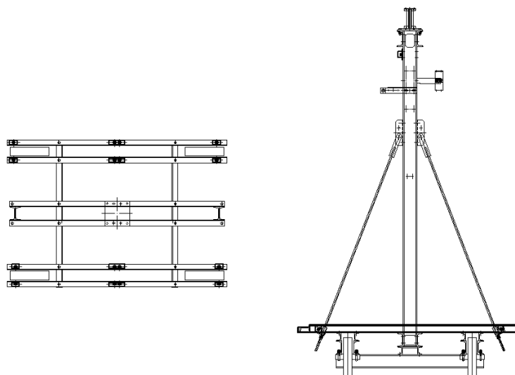
图 11-2 无机房载货电梯（适用于低中吨位）
