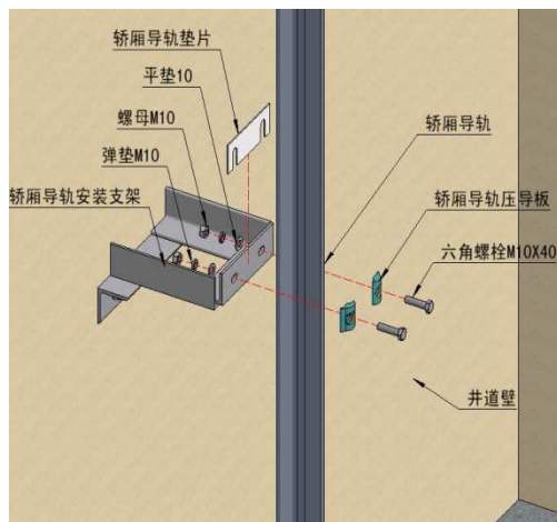
轿厢导轨与导轨支架安装
