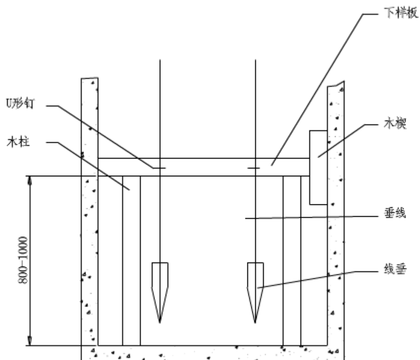
图 5-6 顶层楼板处样板
