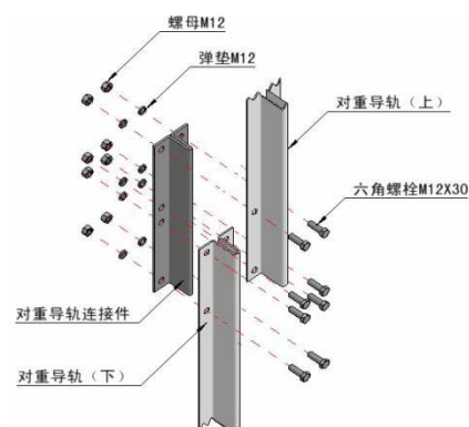
对重导轨对接示意图
